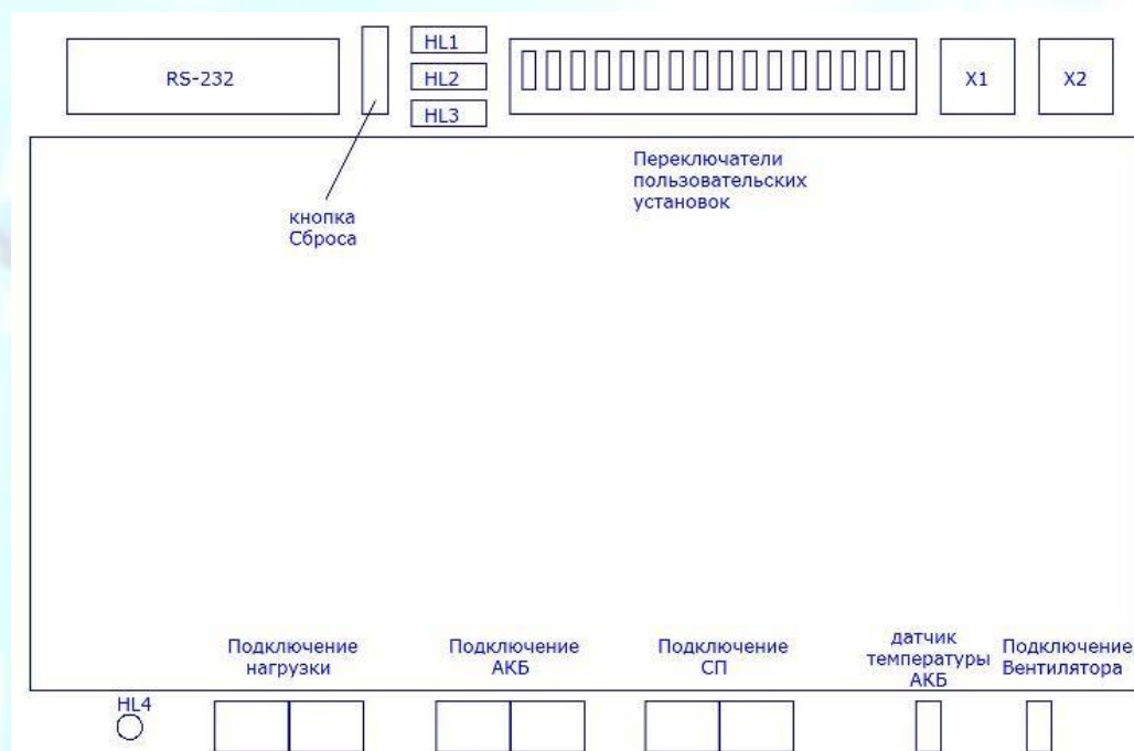
Рис. 1 Органы управления и расположение разъемов.
